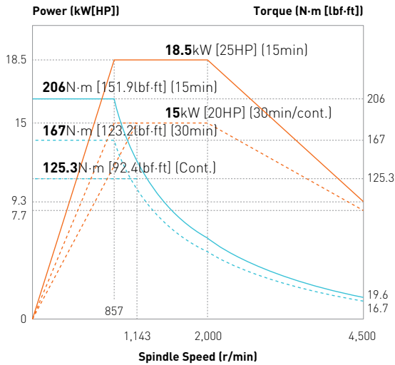
TC22/M 4,500rpm
