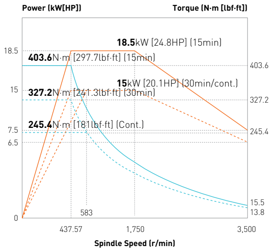
TC22C/MC 3,500rpm
